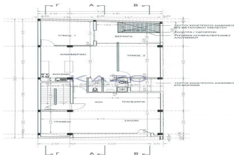
ΚΑΤΟΠΗ Α' ΟΡΟΦΟΥ
