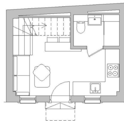
Κάτωψη Ισογείου
