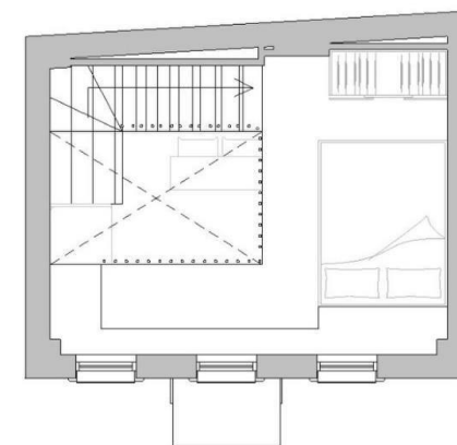
Κάτωψη Μεσοπατώματος
