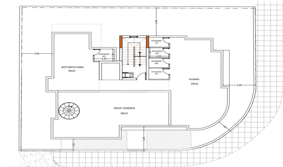
ΚΑΤΟΥΨΗ ΟΡΟΦΗΣ
