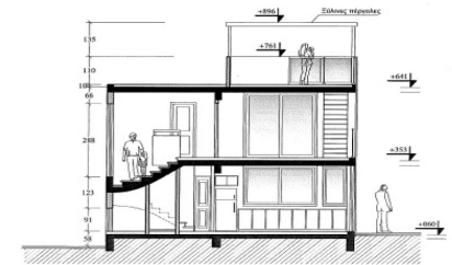
Τομη Α-Α
