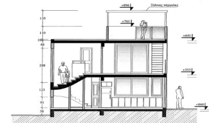
Τομή Α-Α
