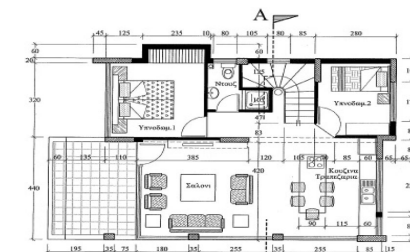
Κατοψη Ισογείου
