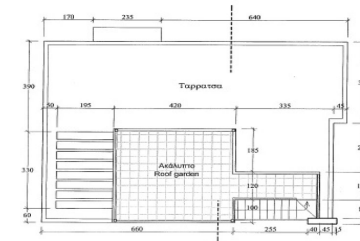
Ανωψη
