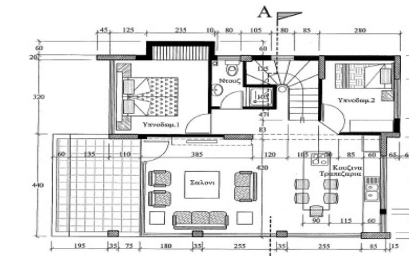
Κατοψη Ισογείου
