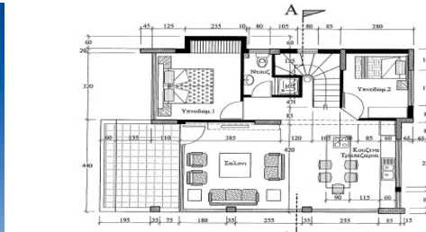
Κατοψη Ισογειου
