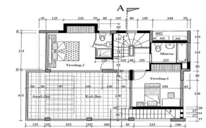
Κατοψη Οροφου
