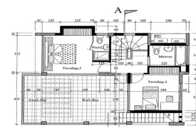
Κατοψη Οροφού
