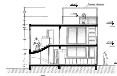
Τομή Α-Α
