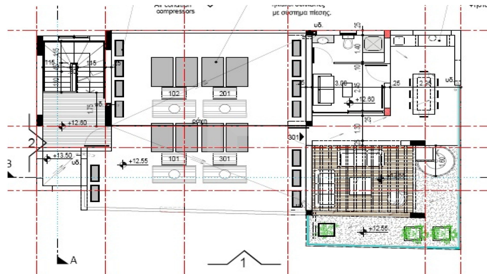
ΚΑΤΟΨΗ ΟΡΟΦΗΣ
