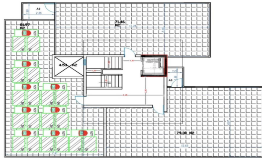
ΚΑΤΟΨΗ ΚΛΗΜΑΚΟΣΤΑΣΕΙΟΥ
