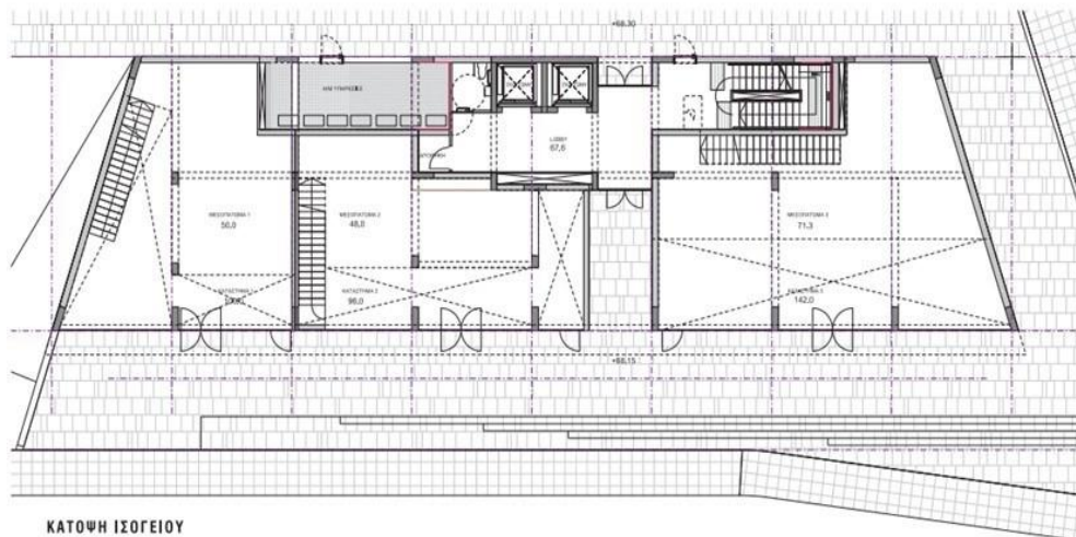
ΚΑΤΩΦΗ ΙΣΟΓΕΙΟΥ ΚΛΙΜΑΚΑ 1:100
