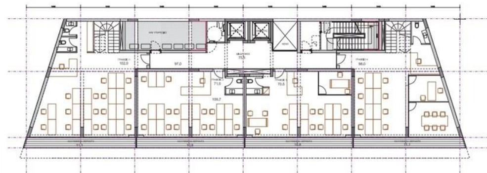
ΚΑΤΩΦΗ ΟΡΟΦΟΥ Κ4 ΚΛΙΜΑΚΑ 1:100
