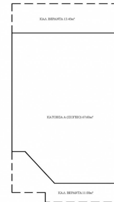
ΕΜΒΑΔΟΜΕΤΡΗΣΗ ΙΣΟΓΕΙΟΥ ΚΑΤΟΙΚΙΑ Α (ΚΑΙΜΑΚΑ 1:200)
