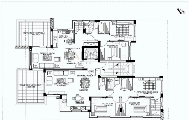
ΚΑΤΟΨΗ 2ου ΟΡΟΦΟΥ
