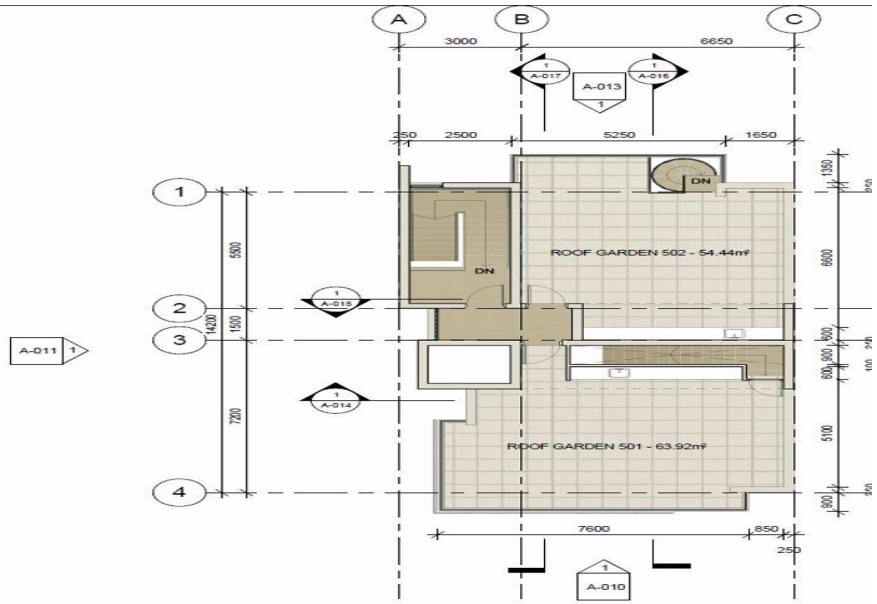
Roof 1 : 100
