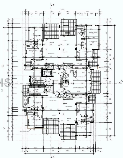
ΚΑΤΩΦΙ ΤΕΤΑΡΤΟΥ ΟΡΟΦΟΥ ΠΟΛΥΚΑΤΟΙΚΙΑ BLOCK A
