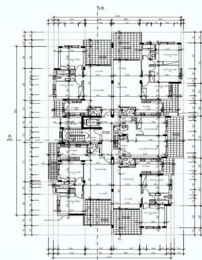
ΚΑΤΩΦΙ ΠΡΩΤΟΥ ΟΡΟΦΟΥ ΠΟΛΥΚΑΤΟΙΚΙΑ BLOCK A
