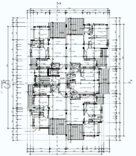
ΚΑΤΩΦΙ ΔΕΥΤΕΡΟΥ ΟΡΟΦΟΥ ΠΟΛΥΚΑΤΟΙΚΙΑ BLOCK A
