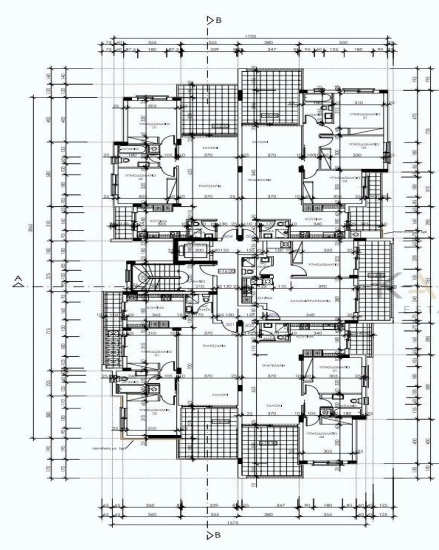
ΚΑΤΟΧΗ ΠΕΜΠΤΟΥ ΟΡΟΦΟΥ ΠΟΛΥΚΑΤΟΙΚΙΑ BLOCK A
