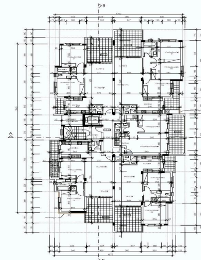
ΚΑΤΩΝ ΠΡΩΤΟΥ ΟΡΟΦΟΥ ΠΟΛΥΚΑΤΟΙΚΙΑ BLOCK A
