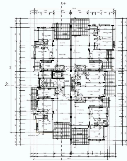
ΚΑΤΟΧΗ ΠΡΩΤΟΥ ΟΡΟΦΟΥ ΠΟΛΥΚΑΤΟΙΚΙΑ BLOCK A
