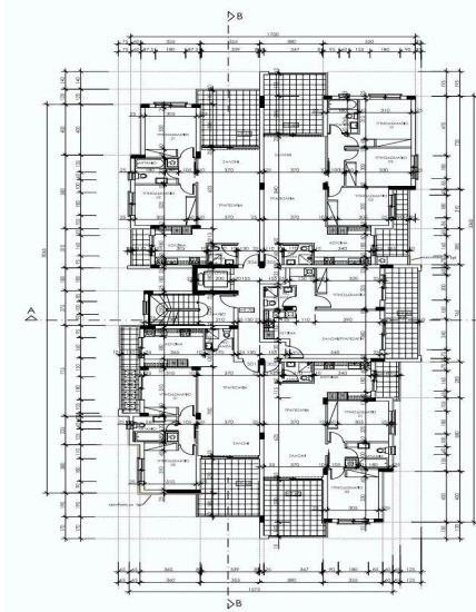
ΚΑΤΟΧΗ ΤΡΙΤΟΥ ΟΡΟΦΟΥ ΠΟΛΥΚΑΤΟΙΚΙΑ BLOCK A
