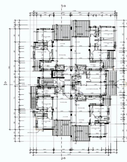
ΚΑΤΩΝ ΠΕΜΠΤΟΥ ΟΡΟΦΟΥ ΠΟΛΥΚΑΤΟΙΚΙΑ BLOCK A
