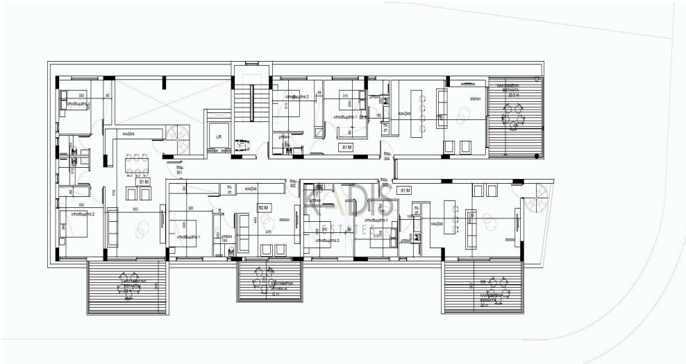
ΚΑΤΑΦΗ 3ου ΟΡΟΦΟΥ
