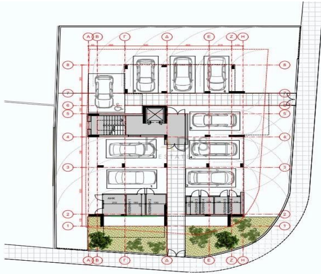
ΚΑΤΩΦΗ ΙΣΟΓΕΙΟΥ
