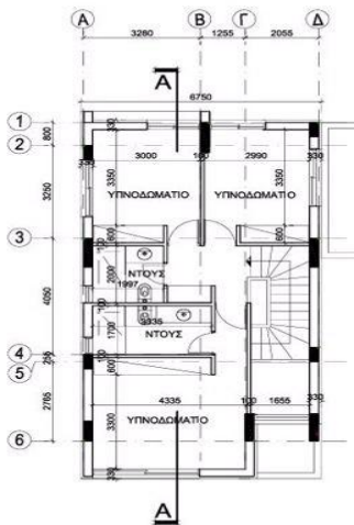
ΚΑΤΟΦΗ ΟΡΟΦΟΥ (ΤΥΠΟΣ Α)
