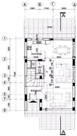
ΚΑΤΟΦΗ ΙΣΟΓΕΙΟΥ (ΤΥΠΟΣ Β)
