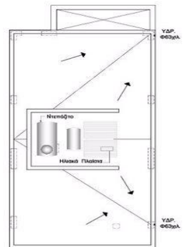
ΚΑΤΟΦΗ ΤΑΡΑΤΣΑΣ
