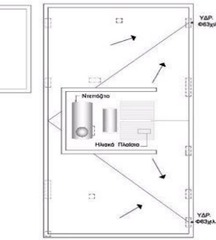
ΚΑΤΟΦΗ ΤΑΡΑΤΣΑΣ (ΤΥΠΟΣ Β)
