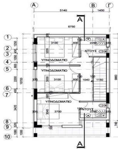
ΚΑΤΟΨΗ ΟΡΟΦΟΥ (ΤΥΠΟΣ Εα)
