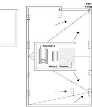
ΚΑΤΟΦΗ ΤΑΡΑΤΣΑΣ
