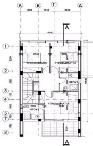
ΚΑΤΟΦΗ ΟΡΟΦΟΥ (ΤΥΠΟΣ Β)
