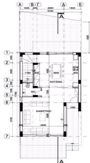
ΚΑΤΟΦΗ ΙΣΟΓΕΙΟΥ (ΤΥΠΟΣ Δα)
