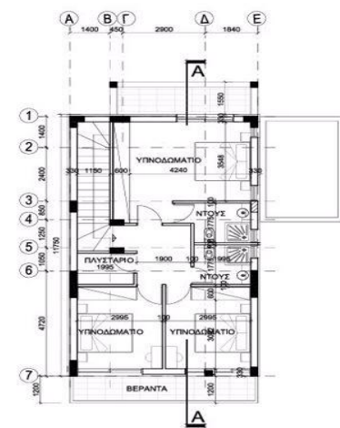
ΚΑΤΟΦΗ ΟΡΟΦΟΥ (ΤΥΠΟΣ Δα)
