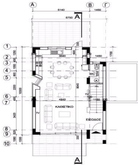
ΚΑΤΟΨΗ ΙΣΟΓΕΙΟΥ (ΤΥΠΟΣ Εα)
