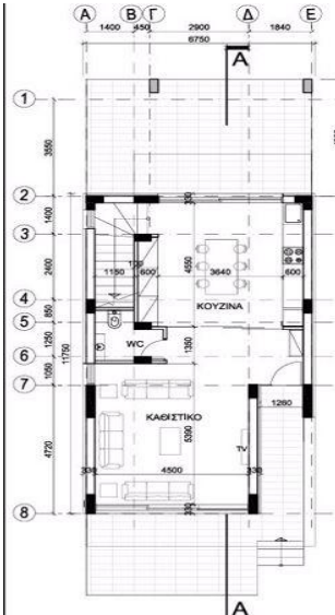
ΚΑΤΟΦΗ ΙΣΟΓΕΙΟΥ (ΤΥΠΟΣ Δ)
