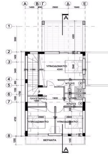
ΚΑΤΟΦΗ ΟΡΟΦΟΥ (ΤΥΠΟΣ Δ)
