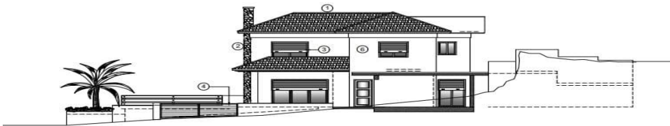
ανατολική όψη
