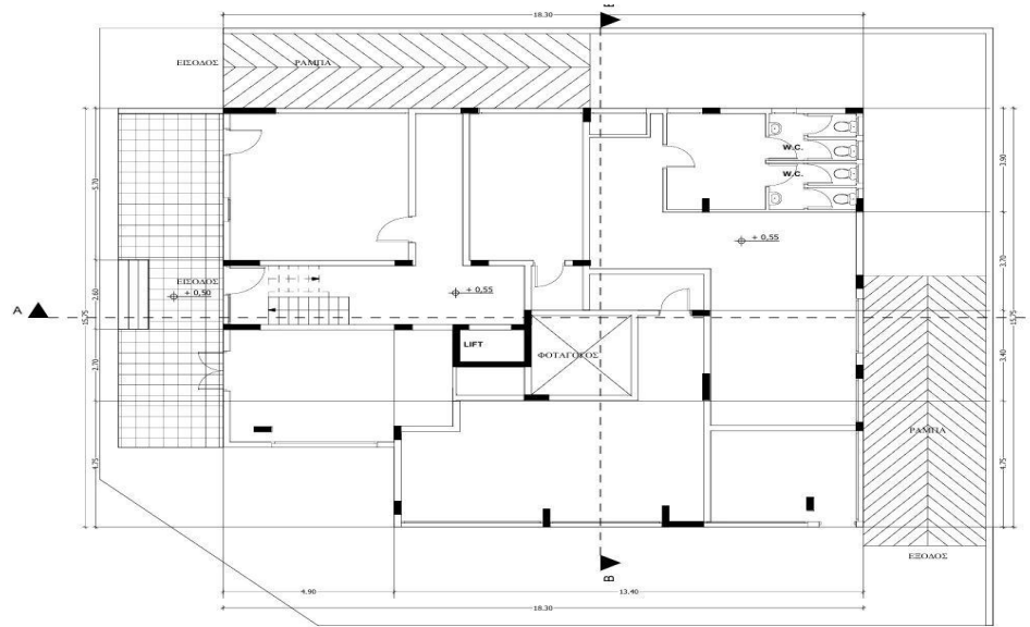
ΚΑΤΟΨΙΣ ΚΑΤΑΣΤΗΜΑΤΩΝ
