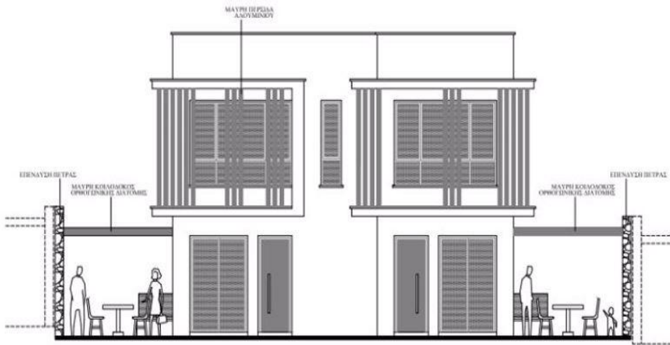
ΝΟΤΙΟΑΝΑΤΟΛΙΚΗ ΟΨΗ-SOUTHEAST ELEVATION
