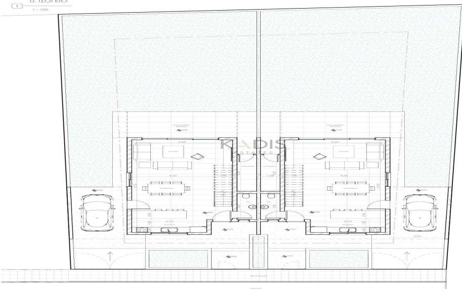
0. ΙΣΟΓΕΙΟ 1:100
