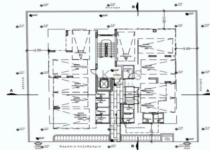
ΚΑΤΟΨΗ ΙΣΟΓΕΙΟΥ ΚΛΙΜΑΚΑ 1:200
