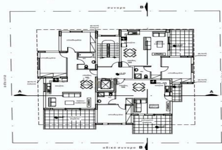
ΚΑΤΟΨΗ 1ΟΥ ΟΡΟΦΟΥ ΚΛΙΜΑΚΑ 1:200
