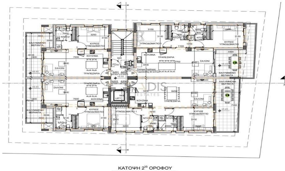
ΚΑΤΟΨΗ 2 ο ΟΡΟΦΟΥ
