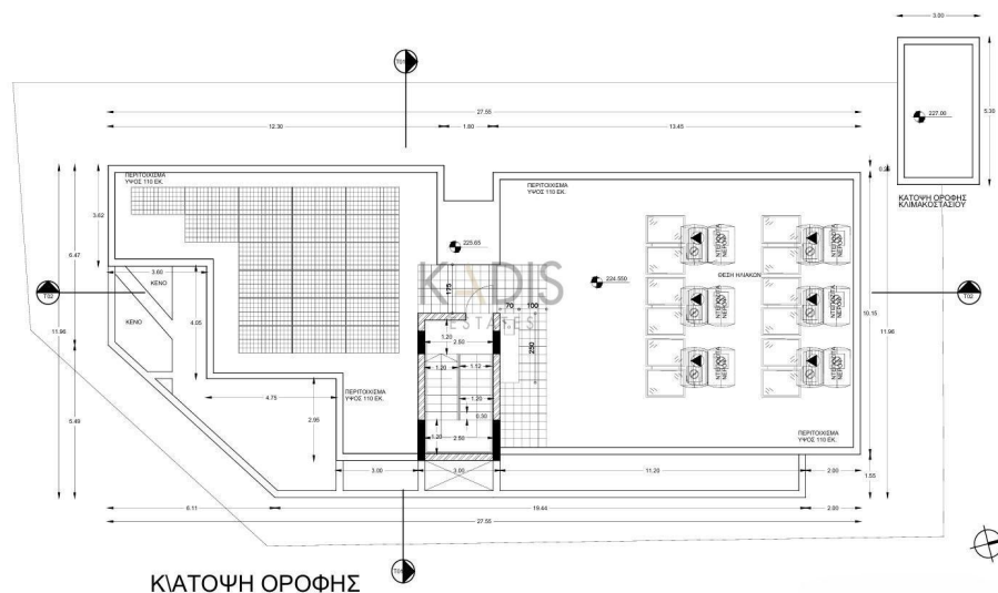
ΚΑΤΟΨΗ ΟΡΟΦΗΣ
