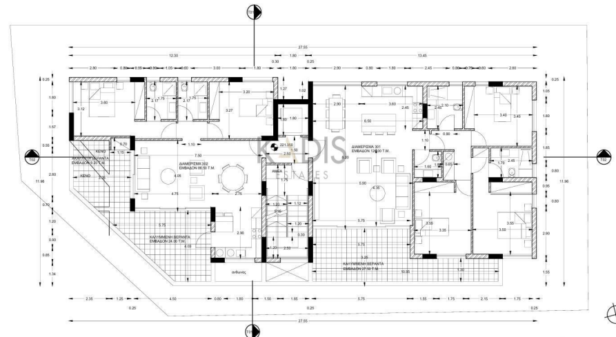
ΚΑΤΩΦΗ 3ΟΥ ΟΡΟΦΟΥ
