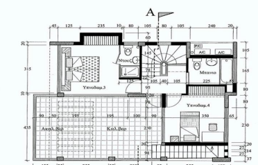
Κατοψη Οροφού
