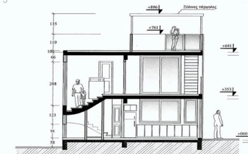
Τομή Α-Α
