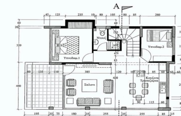
Κατοψη Ισογείου
