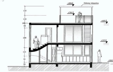
Τομή Α-Α
