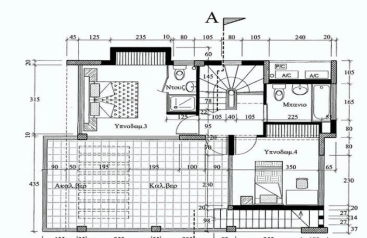
Κατοψη Οροφού
