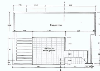
Ανοψη
