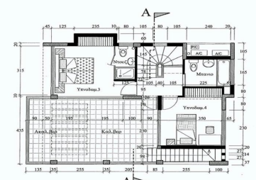
Κατοψη Οροφου
