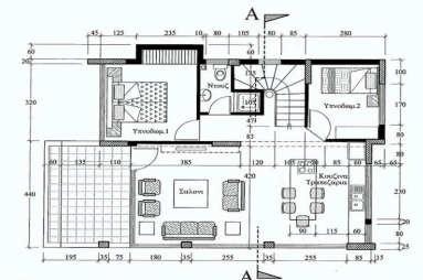
Κατοψη Ισογειου
