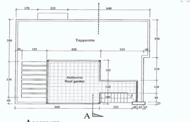
Ανοψη
