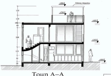
Τομη Α-Α
