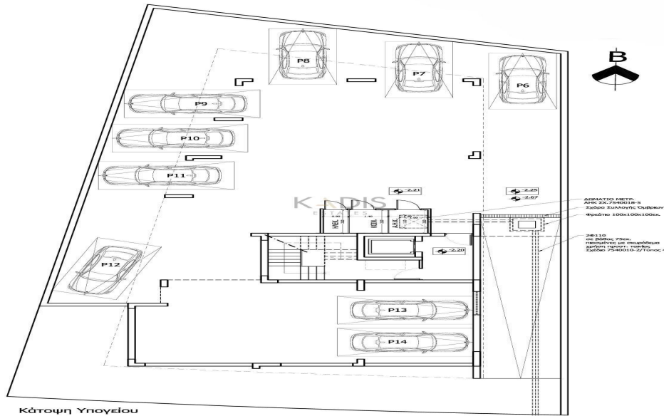
Κάτοψη Υπογείου
