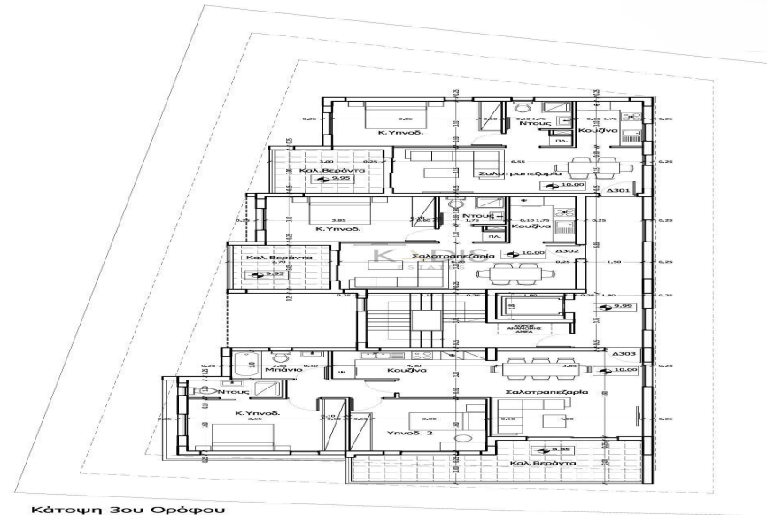
Κάτοψη 3ου Ορόφου
