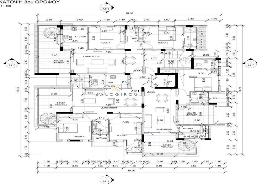
1 ΚΑΤΟΨΗ 3ου ΟΡΟΦΟΥ 1:100
