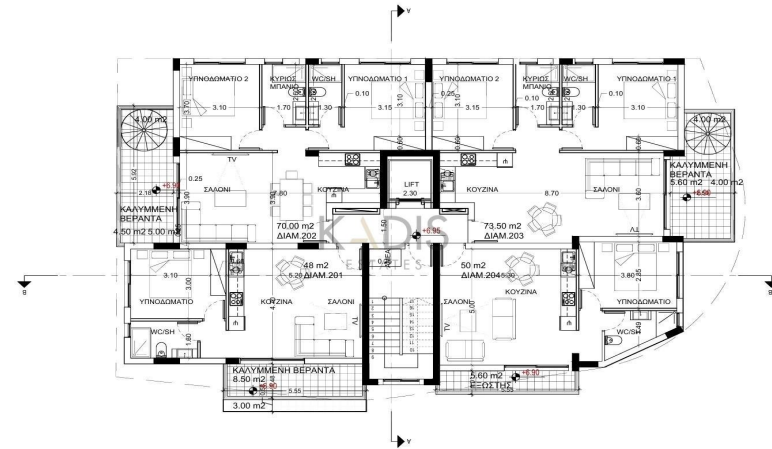
ΚΑΤΟΨΗ 2ΟΥ ΟΡΟΦΟΥ
