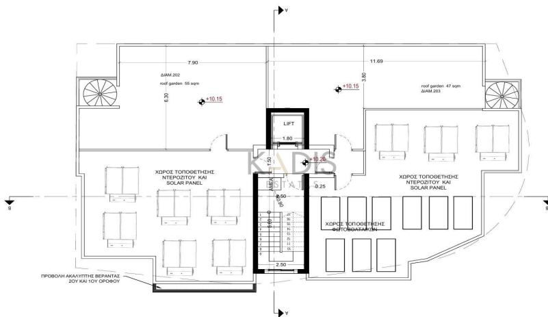
ΚΑΤΟΨΗ ΟΡΟΦΗΣ
