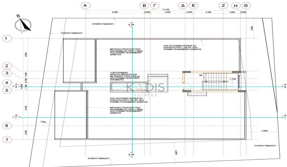
ΚΑΤΟΨΗ ΟΡΟΦΗΣ
