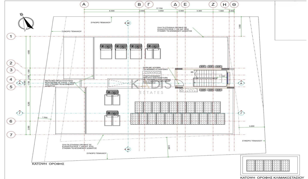
ΚΑΤΟΨΗ ΟΡΟΦΗΣ ΚΑΤΟΨΗ ΟΡΟΦΗΣ ΚΛΙΜΑΚΟΣΤΑΣΙΟΥ
