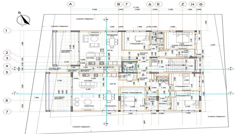
ΚΑΤΟΨΗ 2ΟΥ ΟΡΟΦΟΥ
