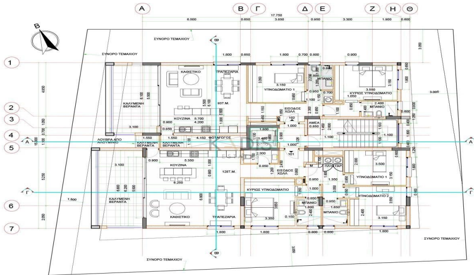
ΚΑΤΟΨΗ 1ΟΥ ΟΡΟΦΟΥ
