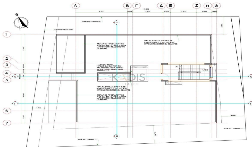
ΚΑΤΟΨΗ ΟΡΟΦΗΣ
