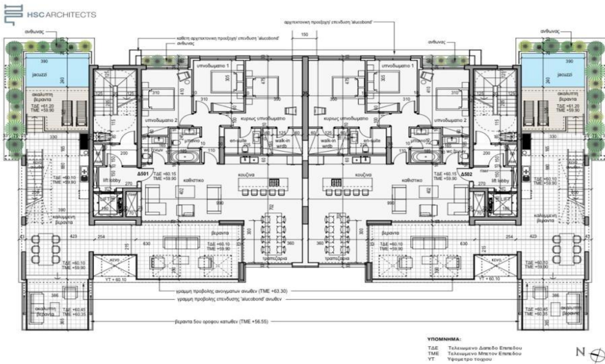
KORONA GARDENS - Αναπτυξη εντος Τεμ. 595, Αγια Ζωνη, Λεμεσος 1: 100 ΚΑΤΟΨΗ ΕΚΤΟΥ ΟΡΟΦΟΥ (PENTHE)
