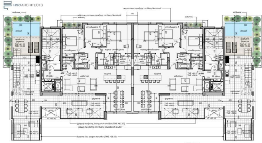
KORONA GARDENS - Αναπτυξη εντος Τεμ. 595, Αγια Ζωνη, Λεμεσος 1: 100 ΚΑΤΟΨΗ ΕΚΤΟΥ ΟΡΟΦΟΥ (PENTH)
