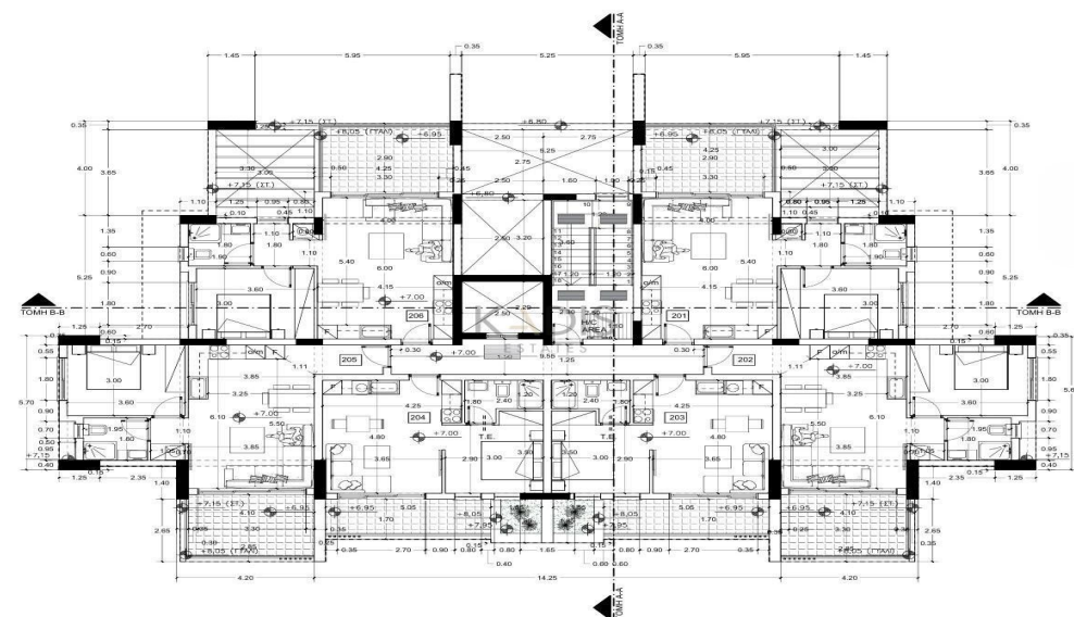
ΚΑΤΟΨΗ Β ΟΡΟΦΟΥ
