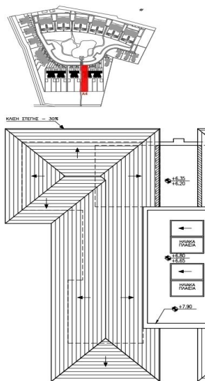
ΚΑΤΟΨΗ ΟΡΟΦΗΣ
