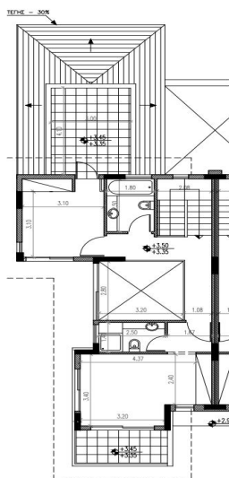
ΚΑΤΟΨΗ ΟΡΟΦΟΥ
