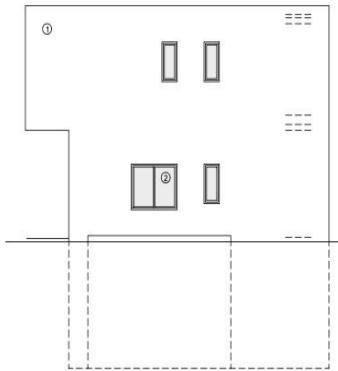
RIGHT ELEVATION
