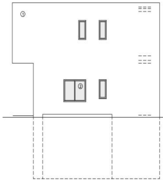
RIGHT ELEVATION
