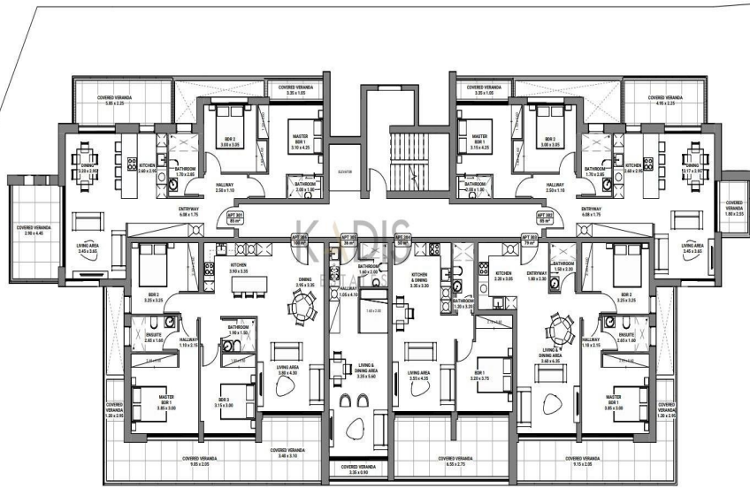
1 Brochure-Third Floor Plan 1 : 100
