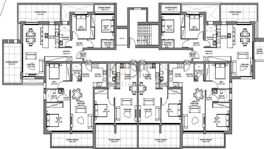
1 Brochure-First Floor Plan 1 : 100
