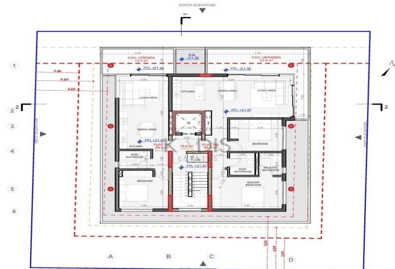
ΠΡΩΤΟΣ ΟΡΟΦΟΣ ΚΛΙΜΑΚΑ 1:200
