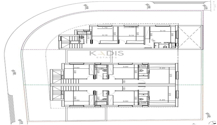
Κατόψεις ορόφου
