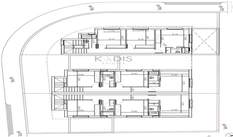
Κατόψεις ορόφου
