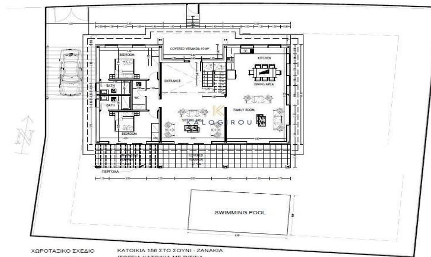
ΧΩΡΟΤΑΞΙΚΟ ΣΧΕΔΙΟ ΚΑΙΜΑΚΑ 1:100
