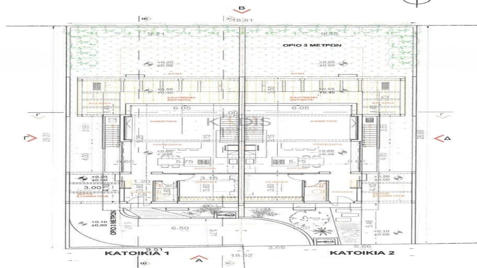
ΧΩΡΟΤΑΞΙΚΟ ΣΧΕΔΙΟ ΚΑΤΩΦΗ ΙΣΟΓΕΙΟΥ ΚΛΙΜΑΚΑ 1:200
