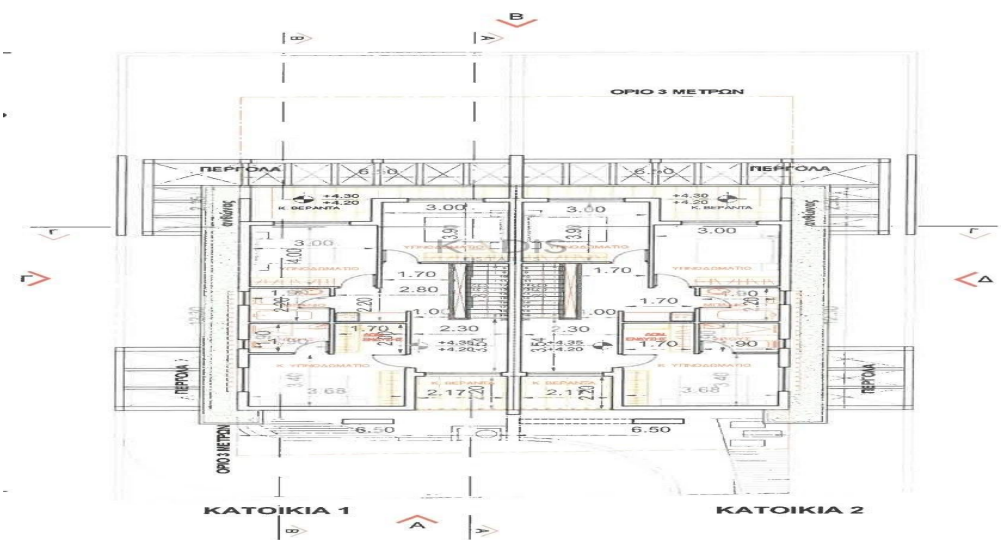
ΚΑΤΩΦΗ ΟΡΟΦΟΥ ΚΛΙΜΑΚΑ 1:200
