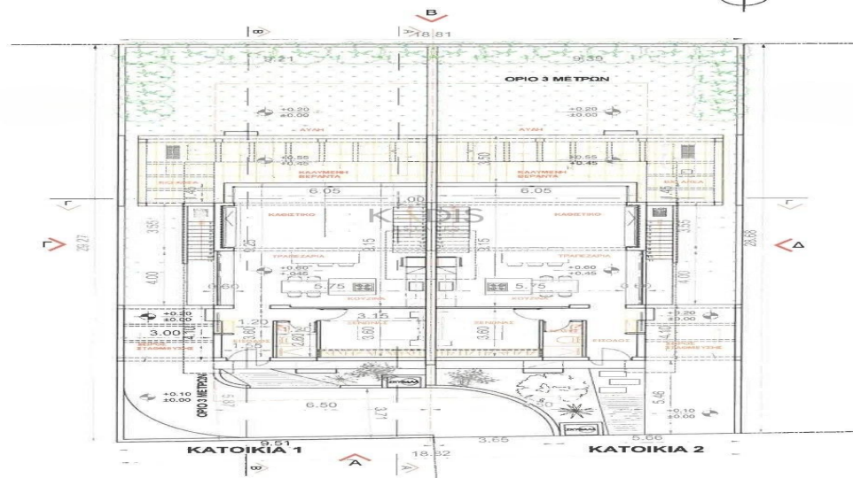
ΧΩΡΟΤΑΞΙΚΟ ΣΧΕΔΙΟ ΚΑΤΟΨΗ ΙΣΟΓΕΙΟΥ ΚΛΙΜΑΚΑ 1:200
