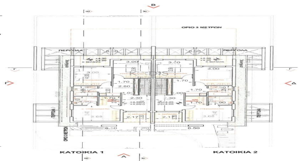
ΚΑΤΩΦΗ ΟΡΟΦΟΥ ΚΛΙΜΑΚΑ 1:200
