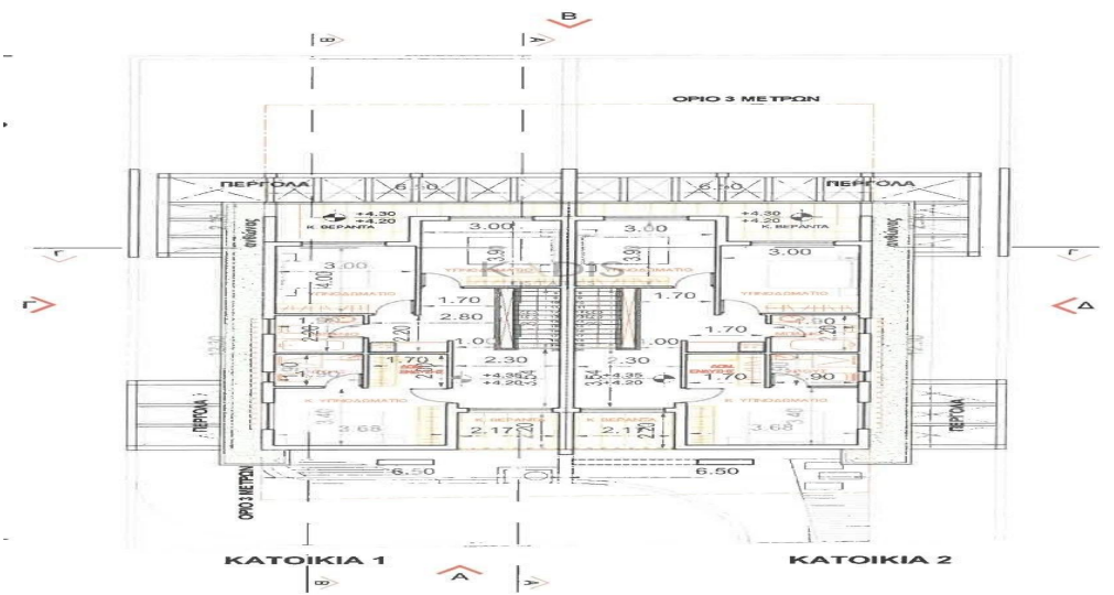
ΚΑΤΟΦΗ ΟΡΟΦΟΥ ΚΛΙΜΑΚΑ 1:200
