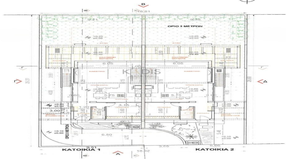
ΧΩΡΟΤΑΞΙΚΟ ΣΧΕΔΙΟ ΚΑΤΟΦΗ ΙΣΟΓΕΙΟΥ ΚΛΙΜΑΚΑ 1:200
