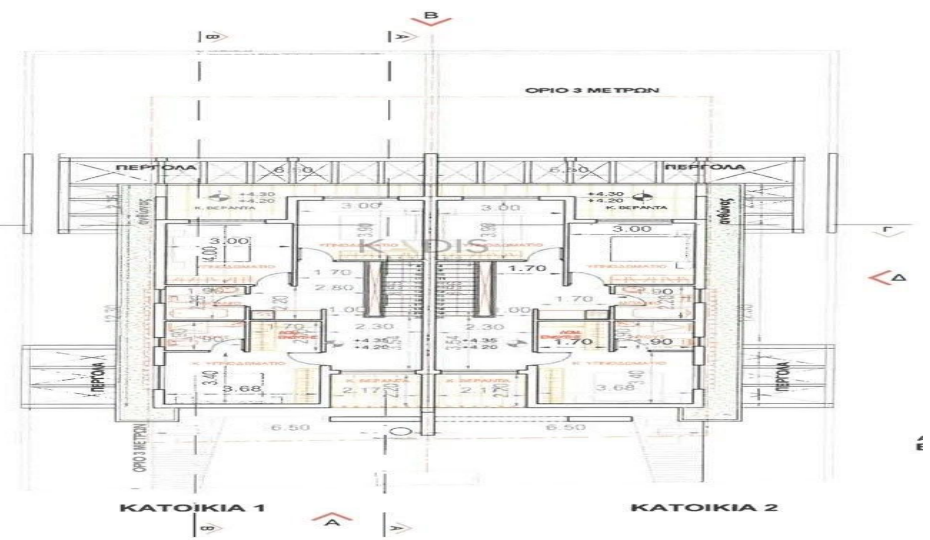
ΚΑΤΟΨΗ ΟΡΟΦΟΥ ΚΛΙΜΑΚΑ 1:200
