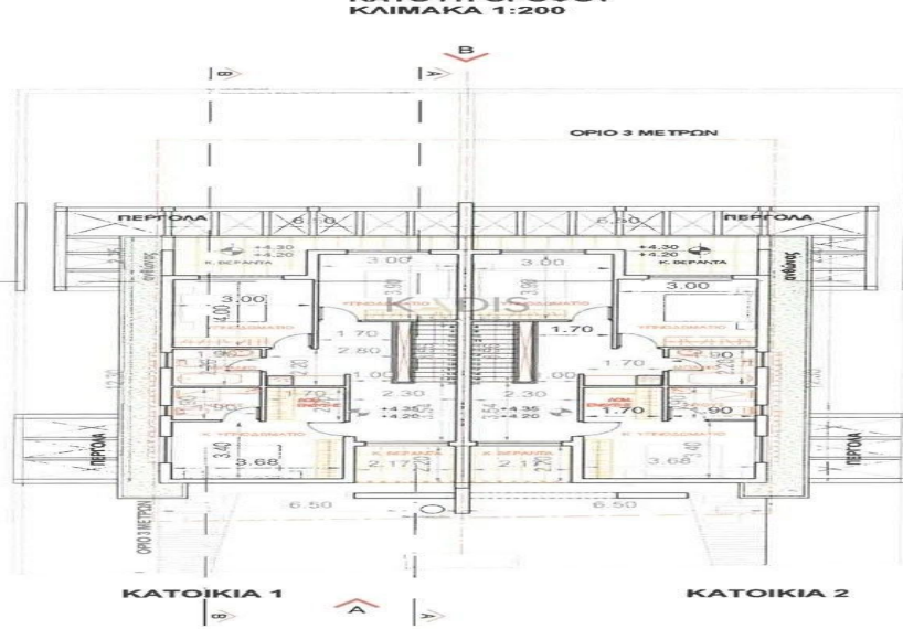
ΚΑΤΟΨΗ ΟΡΟΦΟΥ ΚΛΙΜΑΚΑ 1:200
