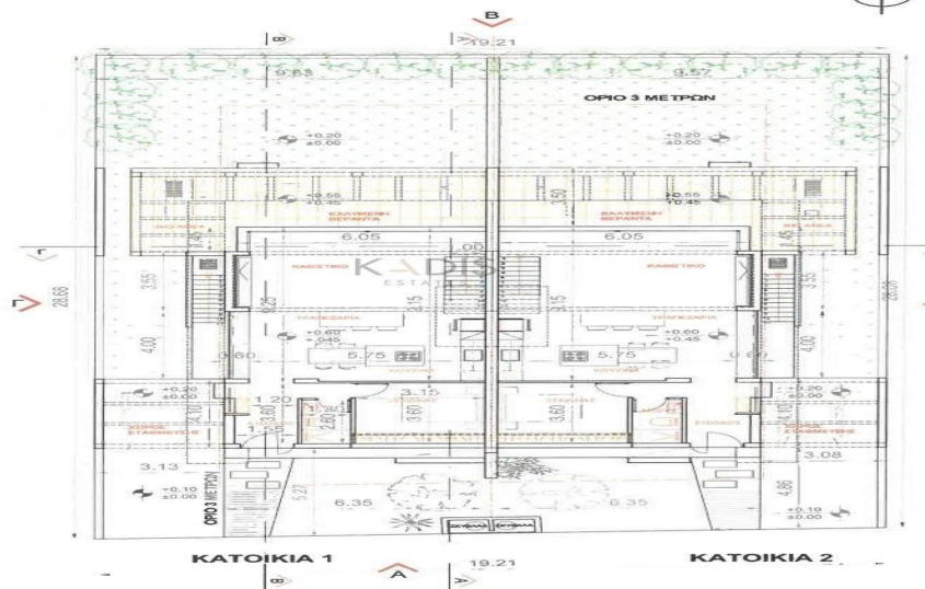
ΧΩΡΟΤΑΞΙΑΚΟ ΣΧΕΔΙΟ ΚΑΤΟΨΗ ΙΣΟΓΕΙΟΥ ΚΛΙΜΑΚΑ 1:200
