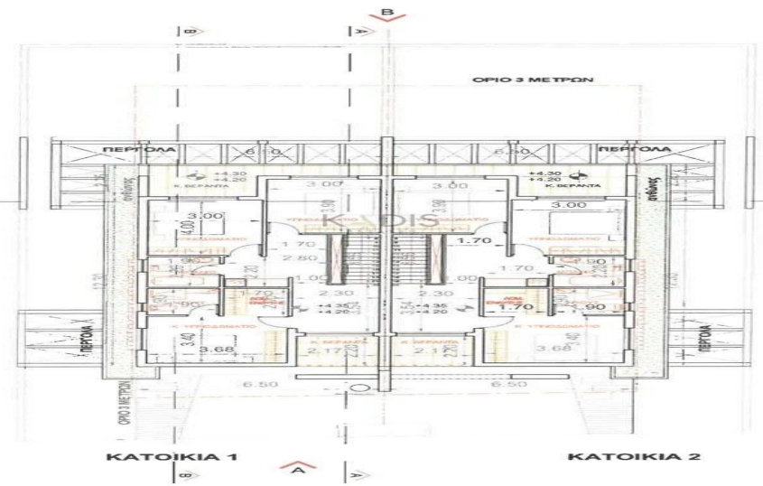
ΚΑΤΟΨΗ ΟΡΟΦΟΥ ΚΛΙΜΑΚΑ 1:200
