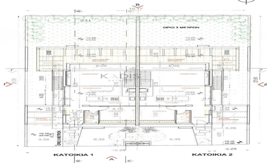
ΧΩΡΟΤΑΞΙΚΟ ΣΧΕΔΙΟ ΚΑΤΟΨΗ ΙΣΟΓΕΙΟΥ ΚΛΙΜΑΚΑ 1:200
