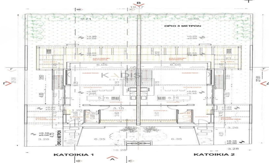
ΧΡΗΣΤΑΙΣΙΚΟ ΣΧΕΔΙΟ ΚΑΤΟΦΗ ΙΣΟΓΕΙΟΥ ΚΛΙΜΑΚΑ 1:200
