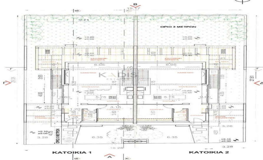
ΧΡΗΣΤΑΞΙΚΟ ΣΧΕΔΙΟ ΚΑΤΟΦΗ ΙΣΟΓΕΙΟΥ ΚΛΙΜΑΚΑ 1:200
