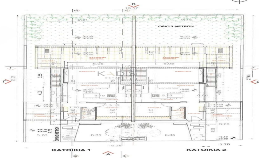
ΧΡΗΣΤΑΙΣΙΚΟ ΣΧΕΔΙΟ ΚΑΤΟΦΗ ΙΣΟΓΕΙΟΥ ΚΛΙΜΑΚΑ 1:200
