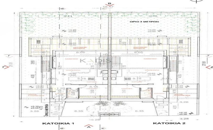
ΧΡΗΣΤΑΣΙΚΟ ΣΧΕΔΙΟ ΚΑΤΟΦΗ ΙΣΟΓΕΙΟΥ ΚΛΙΜΑΚΑ 1:200
