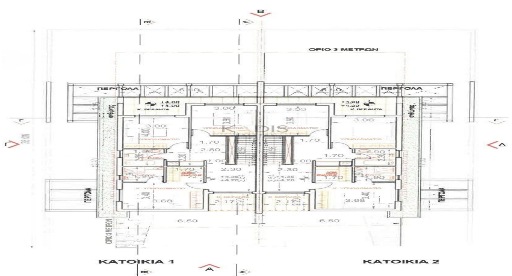
ΚΑΤΟΦΗ ΟΡΟΦΟΥ ΚΛΙΜΑΚΑ 1:200
