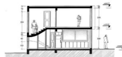
Τομή Α-Α
