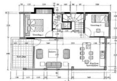
Κατοψη Ισογείου
