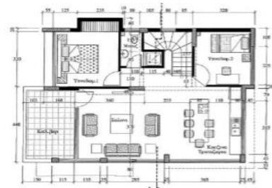
Κατοψη Ισογειου
