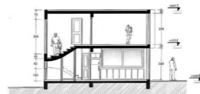
Τομη Α-Α
