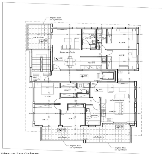
Κάτοψη 3ου Ορόφου Οδικό Δίκτυο
