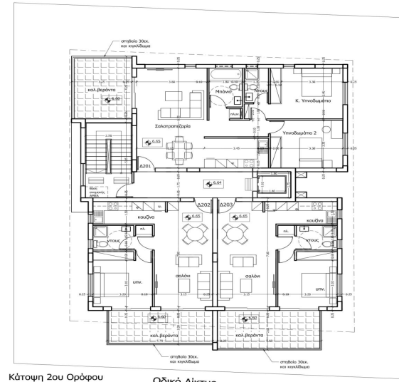
Κάτοψη 2ου Ορόφου Οδικό Δίκτυο
