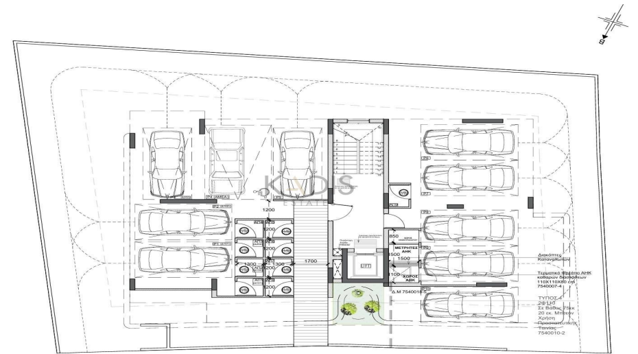
ΚΑΤΟΨΗ ΙΣΟΓΕΙΟΥ
